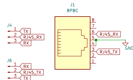
Connecteur RJ45
