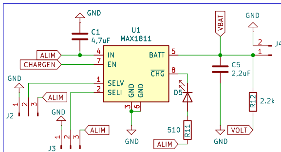
Chargeur LiPo
