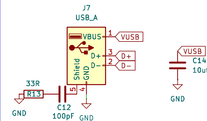
Connecteur USB, mode programmation
