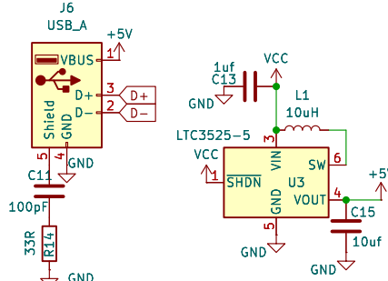
Connecteur USB, mode contrôleur USB
