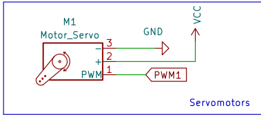
Servomoteurs
